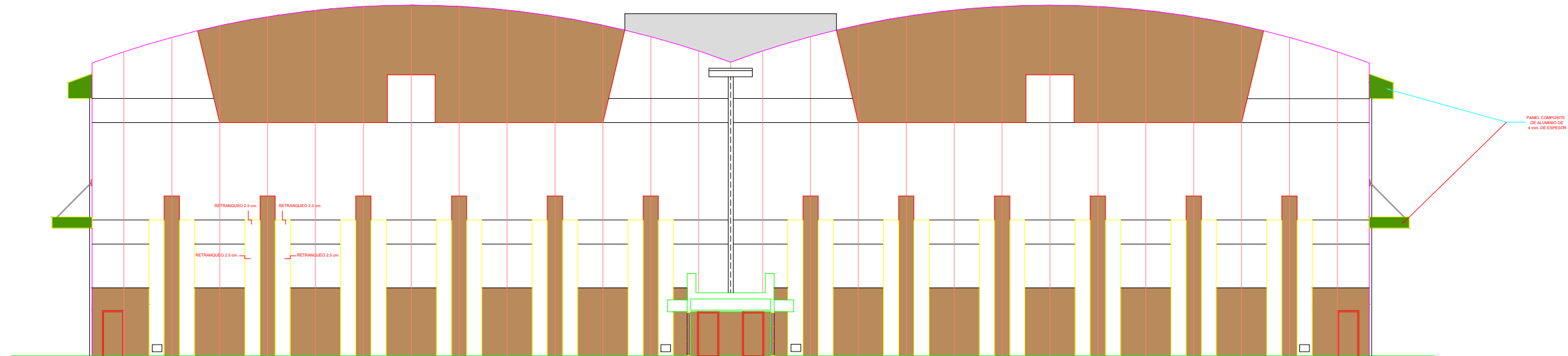
ALZADO 4 PLATO 2A
